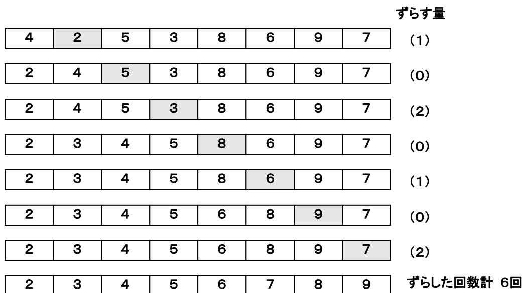
図 6-11 4-ソートおよび2-ソート結果に対して単純挿入法を適用
